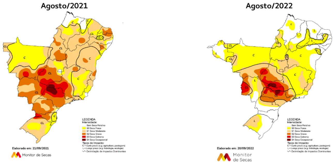
Figura 3 – Seca em agosto de 2021 e agosto de 2022.
